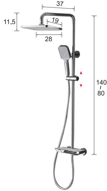
恆溫 ET-SL-333 尺寸：H 80-140 cm 材質：銅鍍鉻
