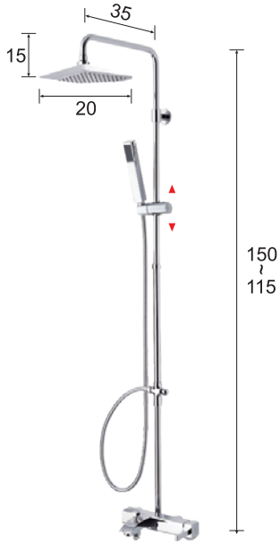
Z-SL-2000-24 尺寸：H 115-150 cm 材質：銅鍍鉻
