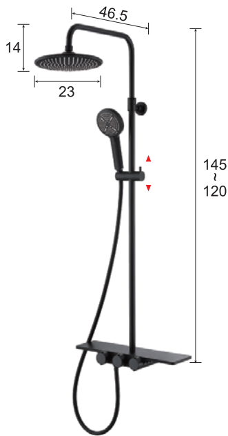
恆溫 Z-109598 尺寸：H 120-145 cm 材質：銅+ABS外殼(消光黑) 備註：冷熱水間距15.2±1.5cm 冷熱出水口需同一水平
